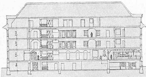
Coupes. — 1 : 600
