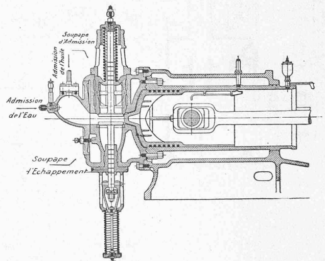
Fig. 4. — Moteur Ruston Proctor .
