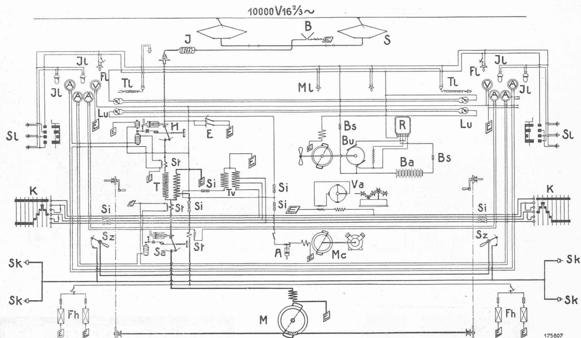
Fig. 15. — Schéma des connexions de la locomotive 1-B-1.
