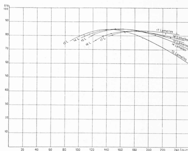
Fig. 8. — Rendement en fonction du nombre de tours pour différentes positions des balais sur le collecteur.
