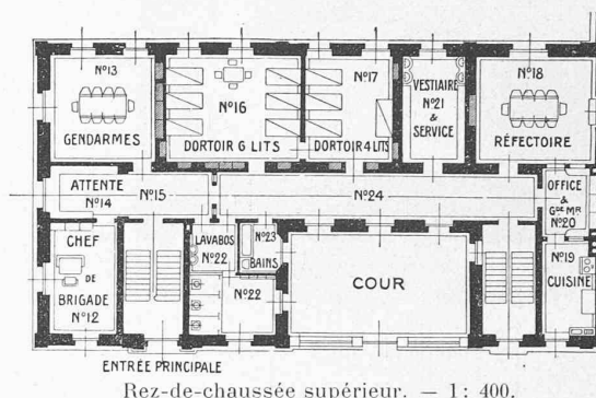
Rez-de-chaussée supérieur. — 1 : 400.
