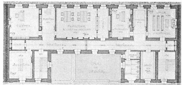
Premier étage. — 1 : 400.
