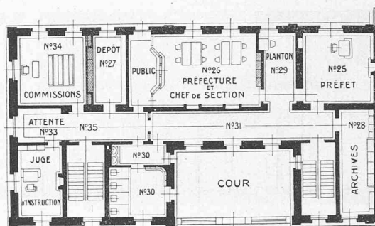
Premier étage. — 1 : 400.
