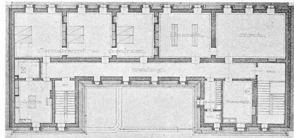
Combles 1 : 400.
