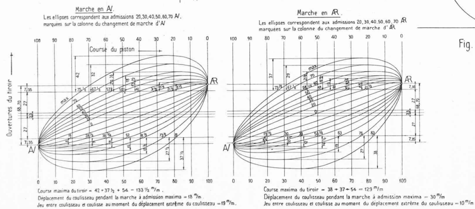
Fig. 59. ELLIPSES POUR DIVERSES ADMISSIONS.
