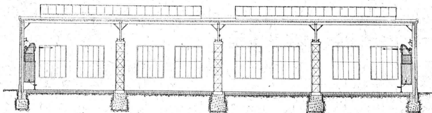
Deux appareils de chauffage Sendric montés dans une fabrique.
