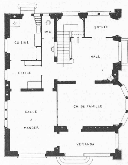
Plan du rez-de-chaussée. — 1 : 200.
