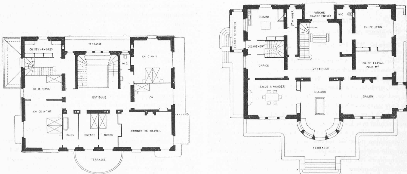
Plans du rez-de-chaussée et de l'étage. — Echelle 1 : 300.
