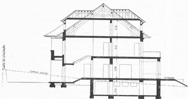
Coupe 1: 300.
