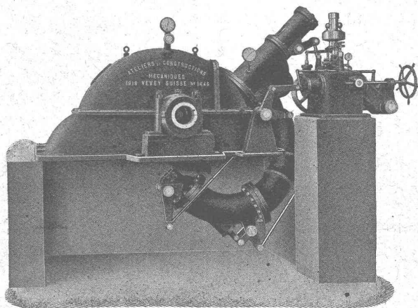
Turbine Pelton avec réglage combiné, 3800 HP. 500 tours.
