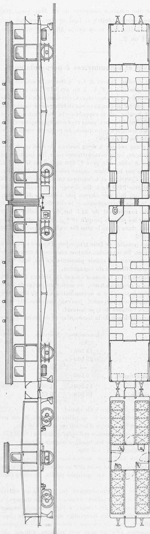
Fig. 1. — Train remorqué par locomotive à accumulateurs type o-c-o. — Projet de la Société Brown, Boveri & Cie. Légende : Batterie d'accumulateurs Tudor de 20 \times 8 = 160 éléments. — Tension moyenne de la batterie : 295 volts. — Capacité pour une décharge unihoraire : 44 amp.-h.; bilhoraire : 331 amp.-h.; trihoraire : 648 amp.-h. — 2 moteurs de traction de 50 HP chacun, à 830 tours/min. ou 80 HP à 630 tours. — Multiplication 4 : 4,93. — Frein à main et à air comprimé. — Locomotive . Longueur entre tampons : 9,5 m.; Rayon des roues : 1040 mm. — Voitures . Longueur entre tampons : 27 m.; rayon des roues : 1040 mm. — Longueur totale du train : 37 m.
