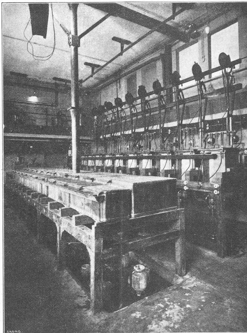
Fig. 6. — Installation pour l'affinage de l'argent.
