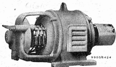
Moteur type MS, avec induit bobiné.
