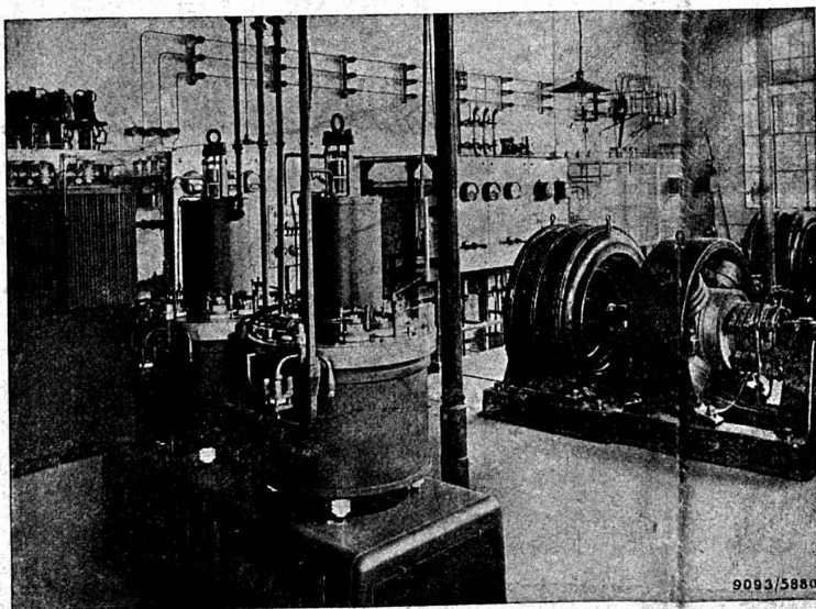
Convertisseurs dans la Salle centrale des Tramways, à Schlieren. Puissance 150 kW. Tension 600 Volts.
