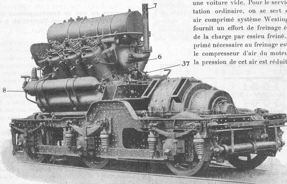
Fig. 3. — Bogie du moteur Diesel avec génératrice et excitatrice accouplées.
