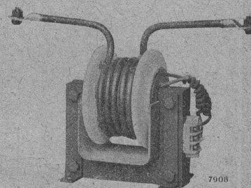
Transformateur d'intensité Type C jusqu'à 200 Amp.
