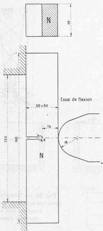
Fig. 25. — Epreuve normale Charpy pour l'essai de flexion par choc.
