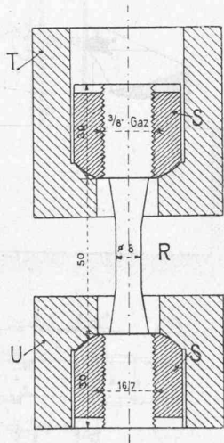
Fig. 25 bis. Epreuve pour l'essai de traction par choc.
