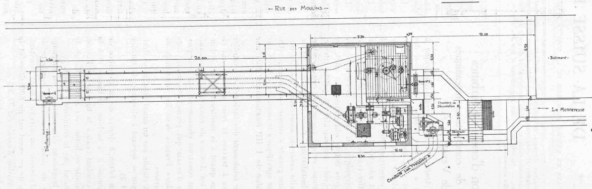
Fig. 1. — Station d'essais des Ateliers de constructions mécaniques de Vevey.
