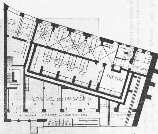
Plan du 1 er sous-sol. — 1 : 800.
