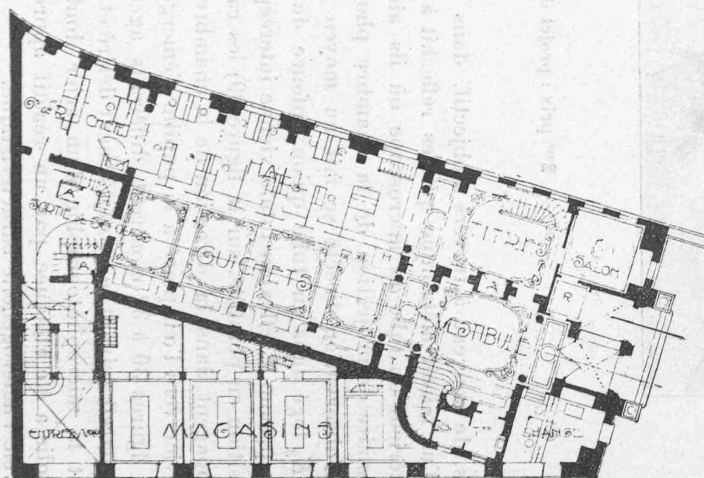
Plan du rez-de-chaussée. — 1 : 800.
