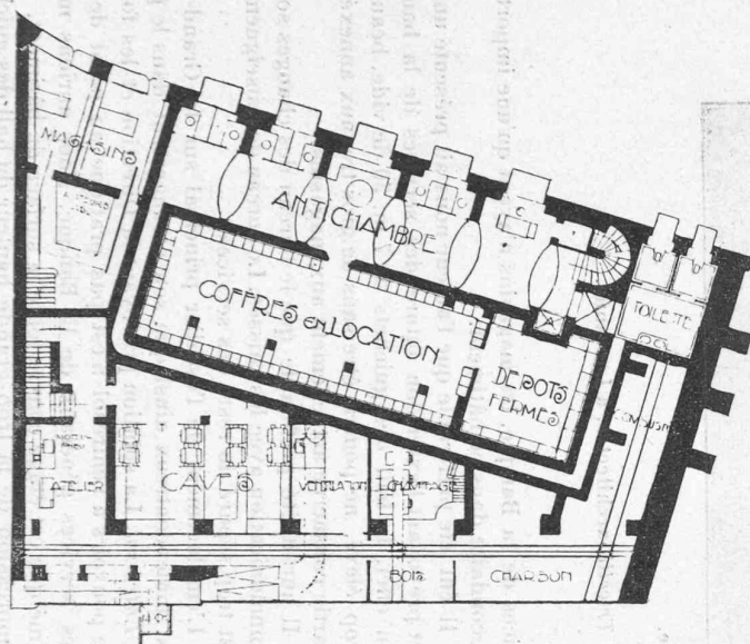
Plan du 2 me sous-sol. — 1 : 800.
