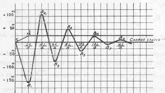
Fig. 14. — Ouverture de cd de v_0 = 0 m à V_f = 4 m,50 en \frac{2L}{a} sec. avec arrêt de la vanne à la fin de la première période.
