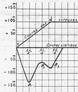
Fig. 16. — Ouverture cd de v_0 = 0 m à V_f = 4 m en 5,33 sec.
