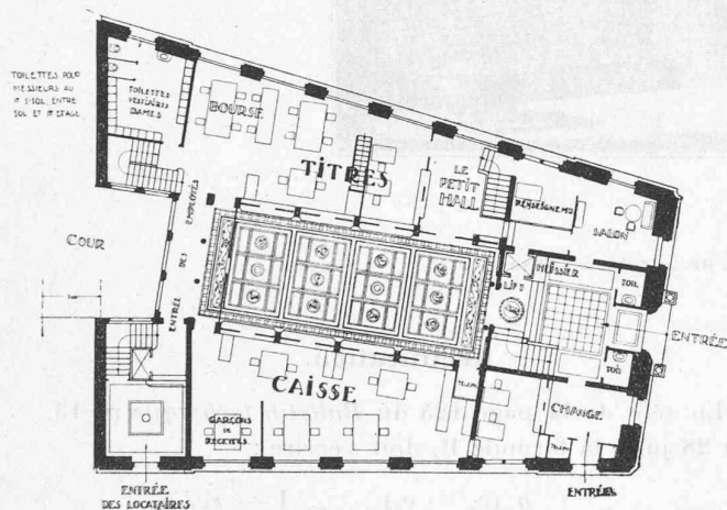
Plan du rez-de-chaussée. — 1 : 800.
