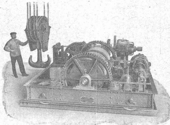
Chariot du pont roulant de 50 tonnes de l'Usine de Ritom (C.F.F.).
