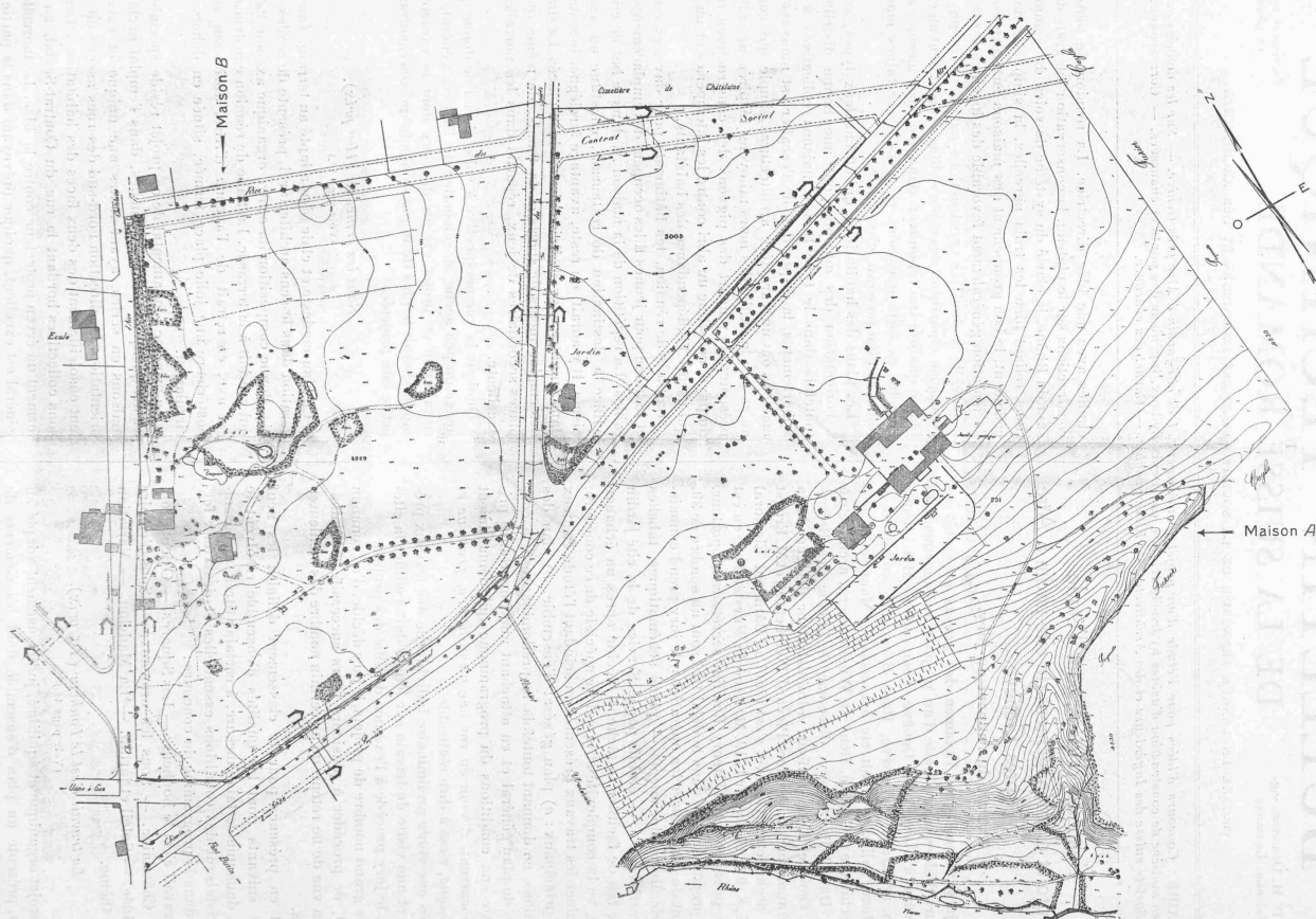
Plan du terrain visé par le concours. — 4 : 3500. Les trois parcelles principales sont indiquées par les nombres : 4929, 3008, 231.
