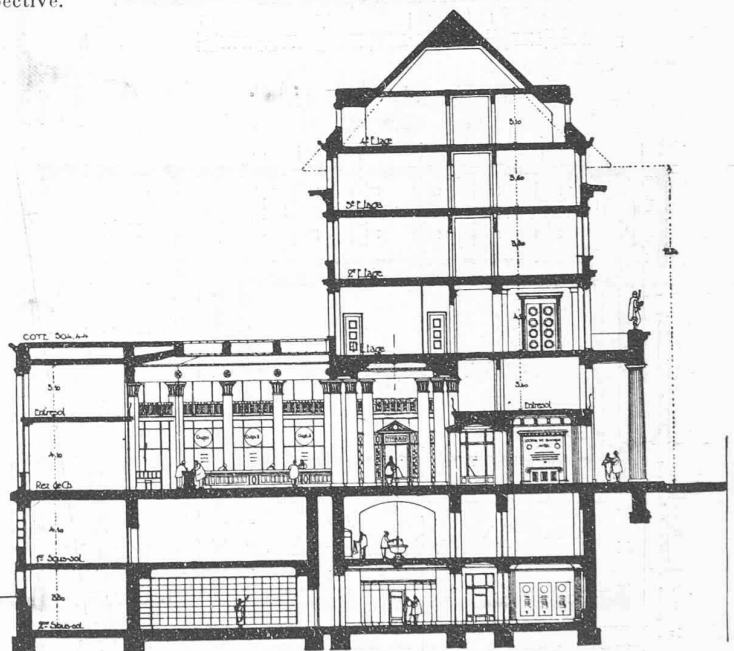
Coupe transversale. — 1 : 400.
