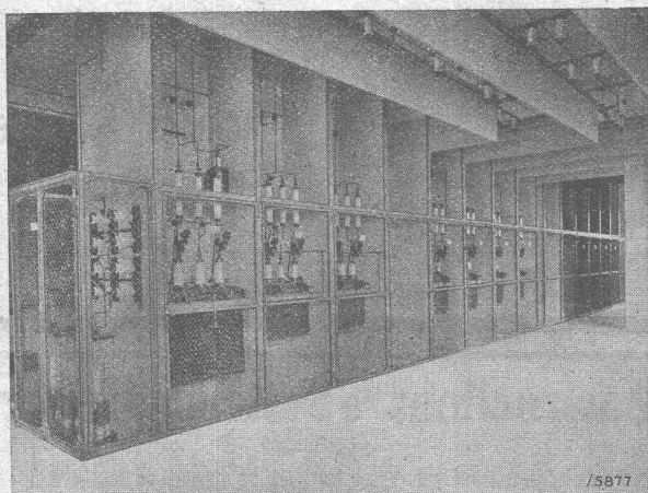
Cellules de distribution de 6500 volts, avec dispositif de protection contre les surtensions (soupapes électriques).
