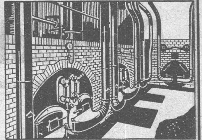
station de soufflerie sous grille « Fehn » pour combustibles pauvres
