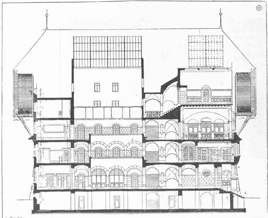
Coupe longitudinale.
