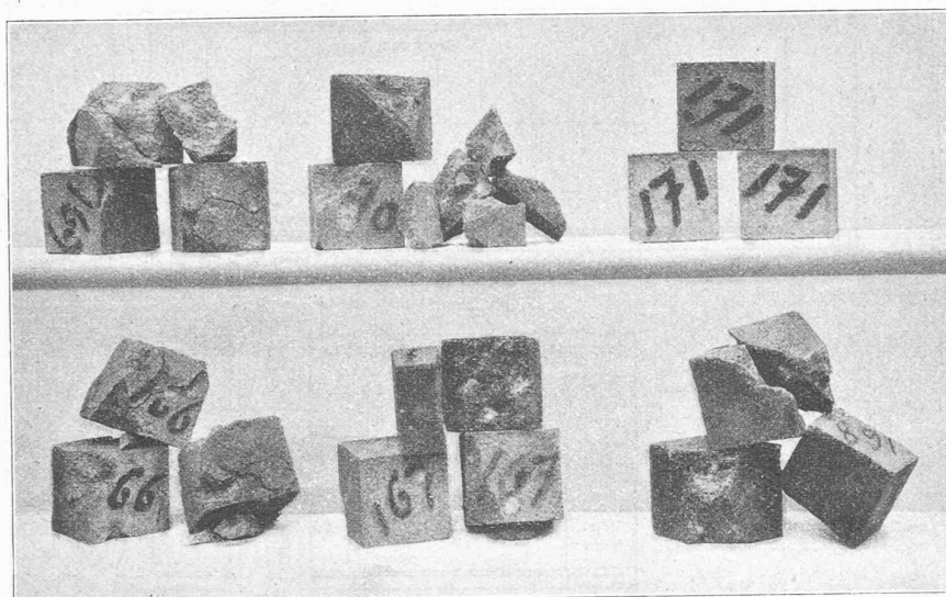
Fig. 1. — Epreuves de béton de scories.
