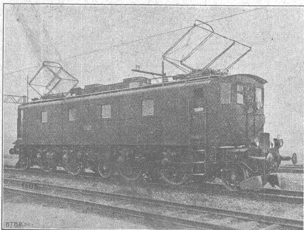
LOCOMOTIVE TYPE «SÉCHERON» IB1 + BI 2400 HP. pour la ligne du Saint-Gothard des Chemins de Fer Fédéraux Suisses.
