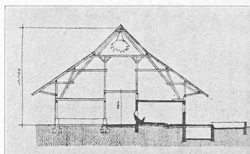
Coupe transversale. — 1 : 400.
