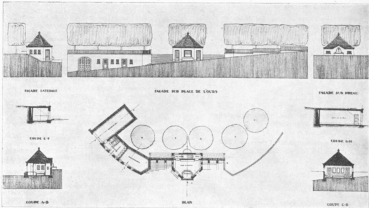
Echelle 1 : 500.
