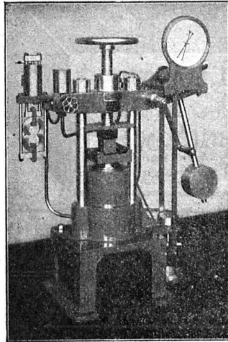
Presse de 30 tonnes pour essais de cubes de ciment.
