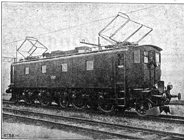
LOCOMOTIVE « SÉCHERON » TYPE IBI + BI 2 400 (HP. pour la ligne du Saint-Gothard des Chemins de Fer Fédéraux Suisses.
