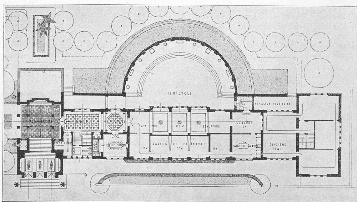
Plan du rez-de-chaussée. — 1 : 500.
