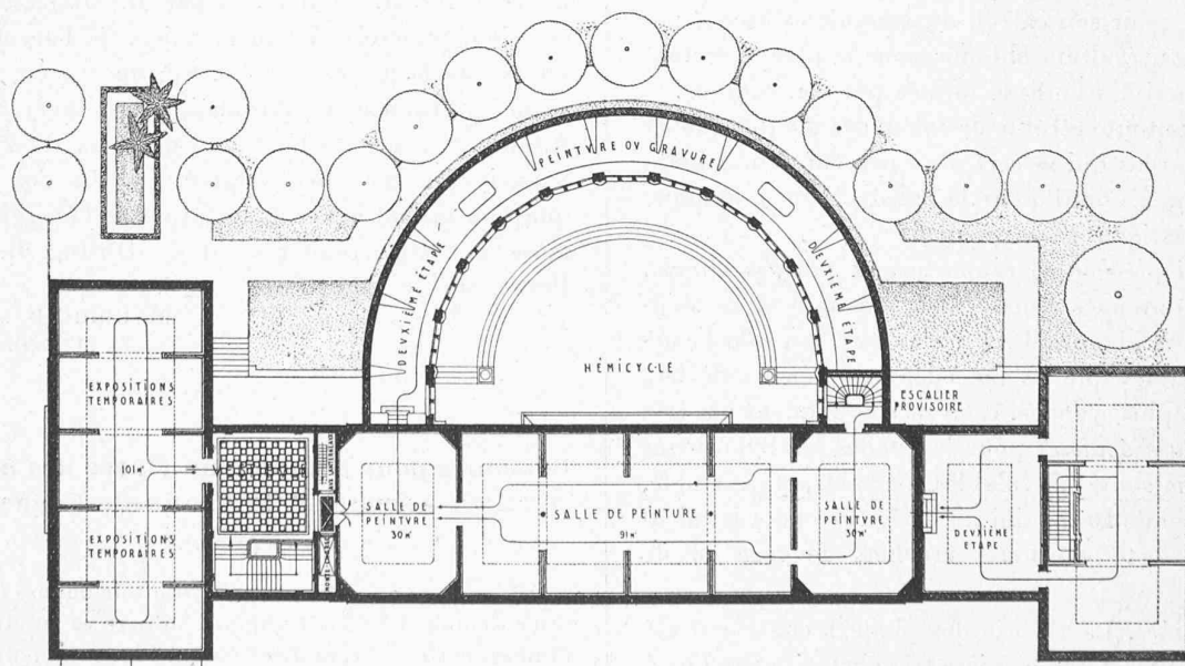
Plan de l'étage. — 1 : 500.
