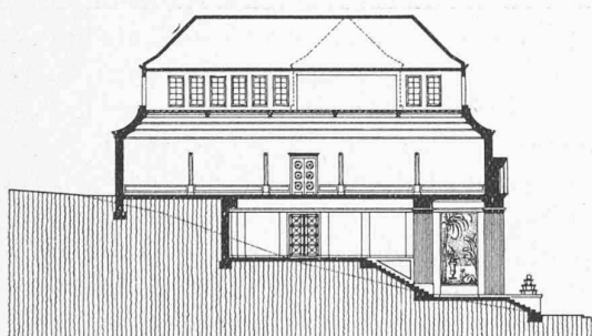
Coupe sur l'entrée. — 1 : 500.
