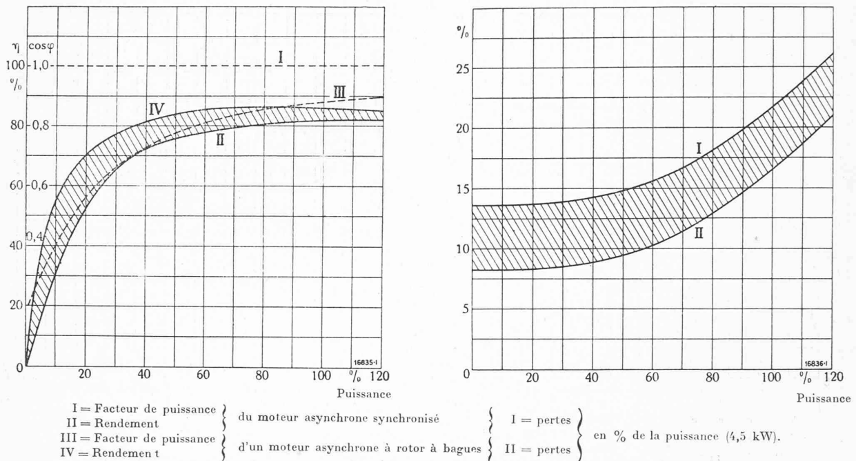
Fig. 7 et 8. — Courbes caractéristiques d'un moteur asynchrone synchronisé avec excitatrice spéciale du type a. Puissance 4,5 kW, 220 volts, 1500 t/min, 50 pér/sec.
