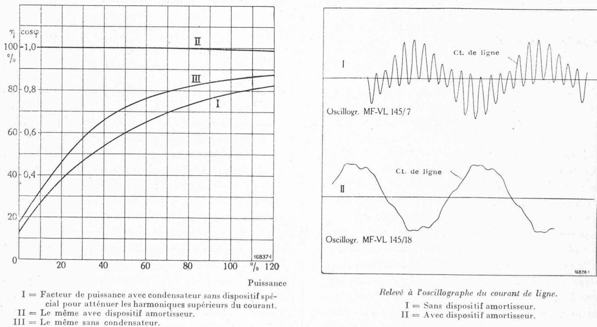
Fig. 9 et 10. — Courbes caractéristiques d'un moteur asynchrone avec ou sans couplage en parallèle d'un condensateur statique du type b. Puissance 2,2 kW, 220 volts, 1500 t/min, 50 pér/sec; capacité de la batterie = 23 \mu F environ.
