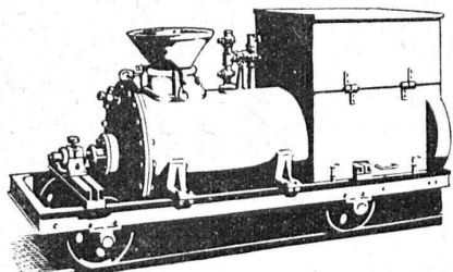
Machine à injection de ciment.
