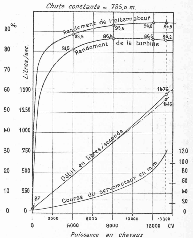
Fig. 14. — Caractéristiques de la turbine II de Ritom (1923).
