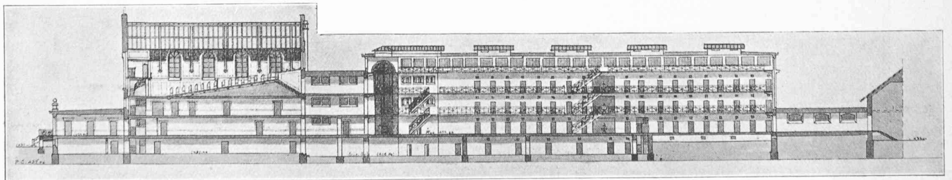
Coupe longitudinale. — 1 : 800.
