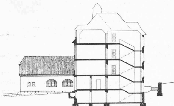
Coupe transversale. — 1 : 500.
