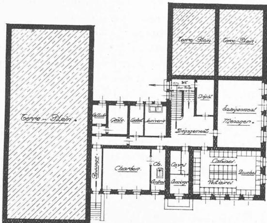
Plan du sous-sol. — 1 : 500.
