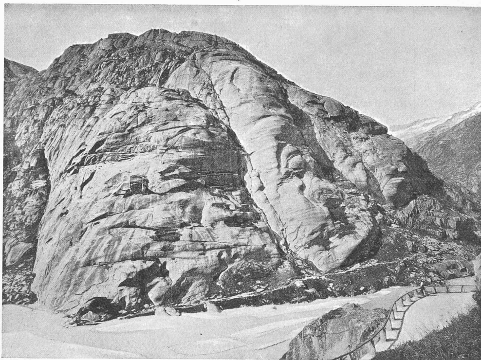
Fig. 14. — Entrée de la Spittallamm; flanc gauche de la gorge.
