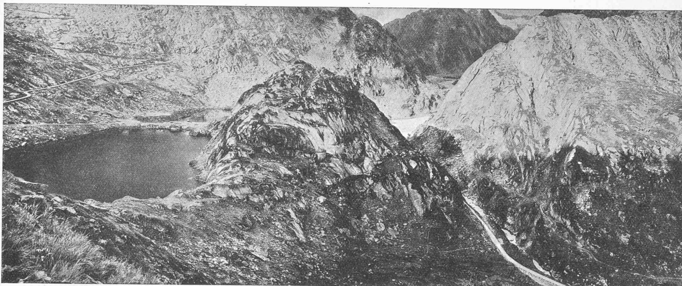
Fig. 12. — Vue du Grimsel, prise du nord-est. A gauche, lacs actuels; en avant de ceux-ci, la barre de la Seeuferegg, au centre, le Nollen et à droite, la gorge de la Spitallamm.
