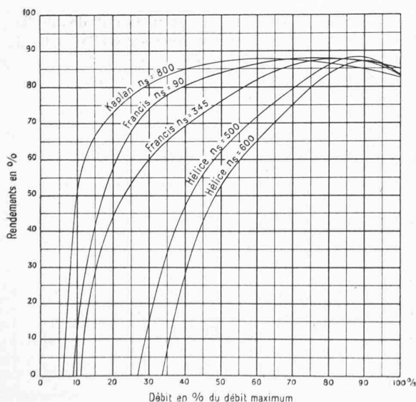
Fig. 6 et 7. — Rendements en fonction : 1 o de la puissance et 2 o du débit, de différents types de turbines Voith .
