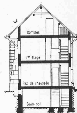
Coupe sur E.
