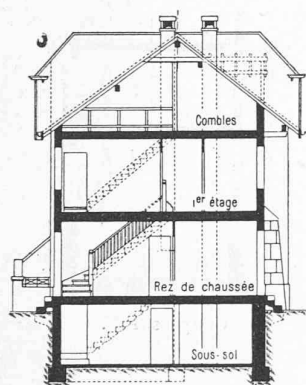
Coupe sur D'.
