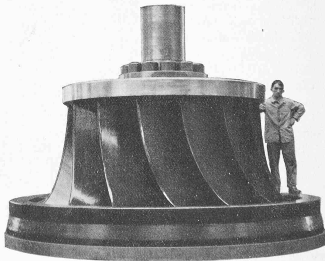
Fig. 3. — Roue d'une des turbines de Parahyba (Brésil). H = 31,7 m. ; Q = 91,3 m 3 /sec. ; N = 32\,500 ch. ; n = 125 t./min.
