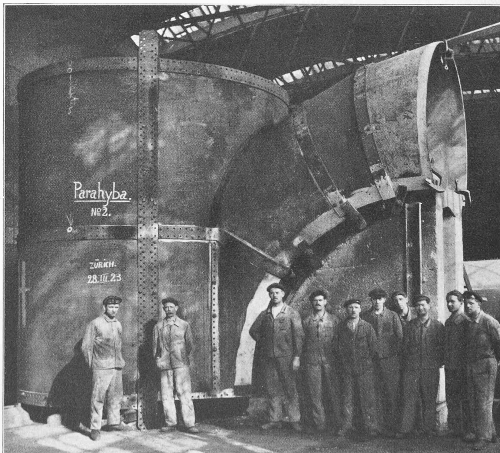
Fig. 1. — Collecteur et tronçon de bêche spirale de l'usine de Parahyba (Brésil). H = 31,7 \text{ m.} ; Q = 91,3 \text{ m}^3/\text{sec.} ; N = 32\,500 \text{ ch.} ; n = 125 \text{ t/min.}
