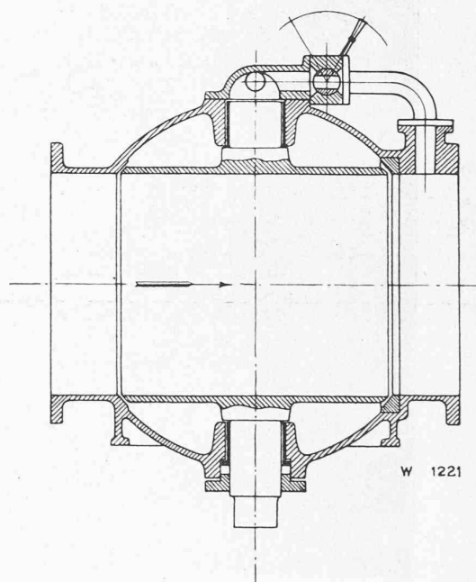
Fig. 7. — Position d'ouverture
