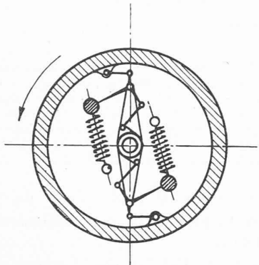
Fig. 2. — Régulateur d'inertie.
