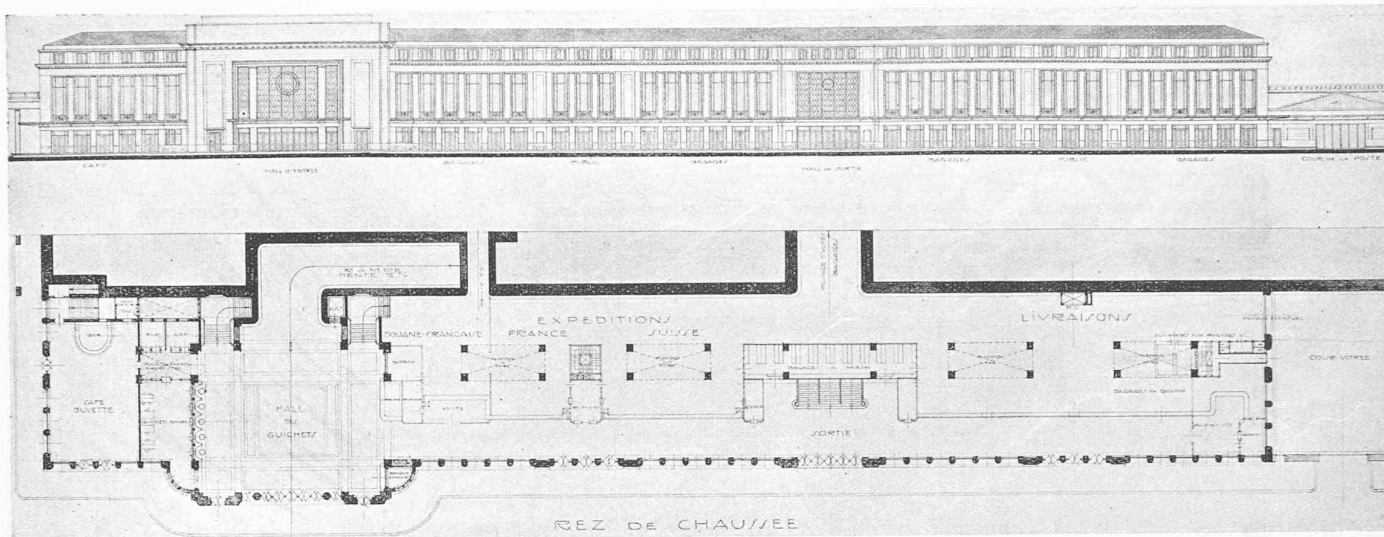
Facade principale et plan du rez-de-chaussée. — 1 : 1000.
