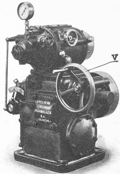
Fig. 5. — Régulateur de 100 kgm.
