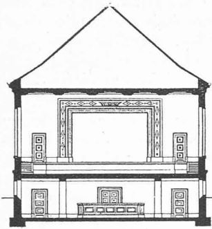
Coupe transversale.
