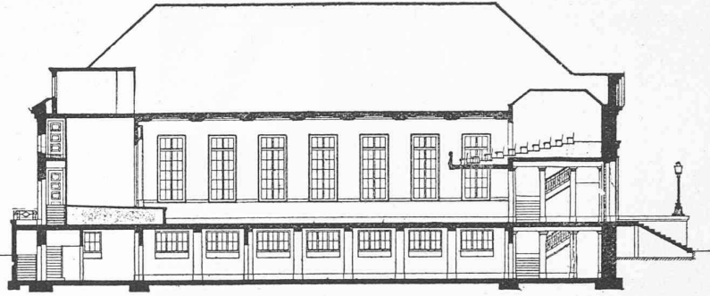
Coupe longitudinale.
