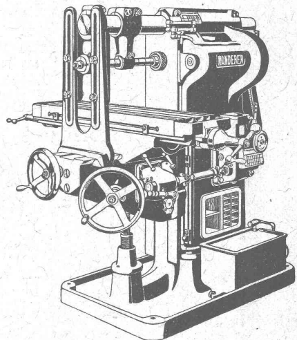
FRAISEUSE - WANDERER
