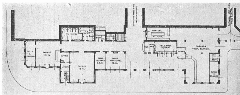
Plan du rez-de-chaussée. — 1 : 800.
