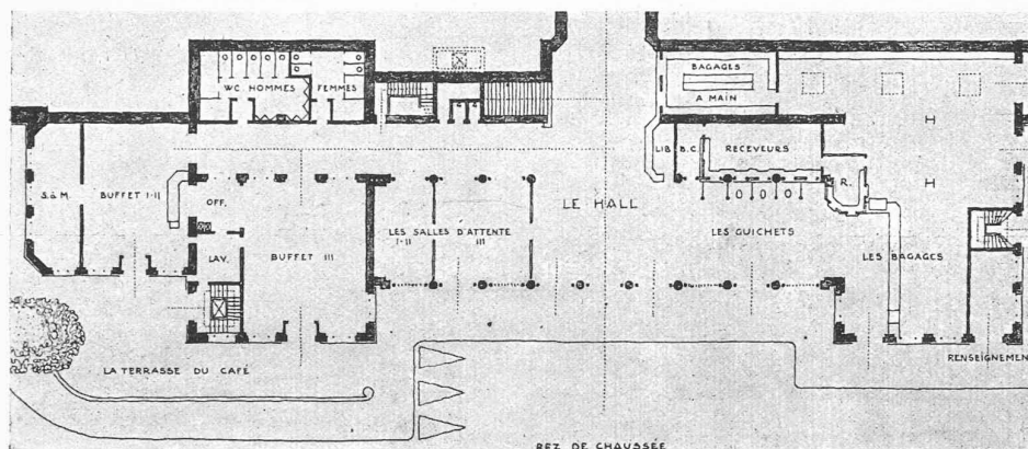
Plan du rez-de-chaussée. — 1 : 600.
