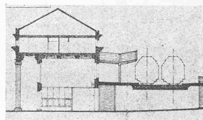
Coupe à travers le hall.
