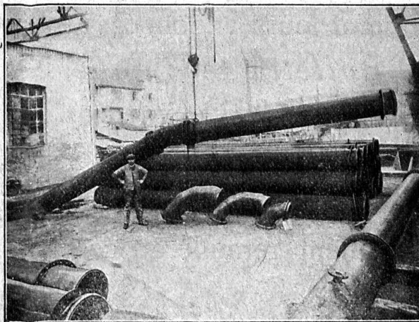
Conduite de 500 mm. de diamètre, en tôle entièrement soudée à l'arc électrique. — Pression en service : 140 m. d'eau.
